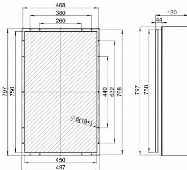
ЧЕРТЕЖИ ПРИСОЕДИНИТЕЛЬНЫХ РАЗМЕРОВ UNISPLIT NS-1500(1)W
