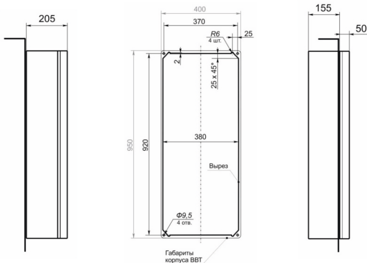
Монтажный вырез утопленный монтаж
