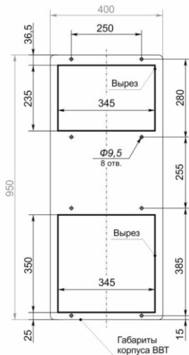
Монтажный вырез наружный монтаж
