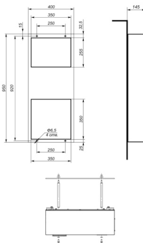
МОНТАЖНЫЙ ВЫРЕЗ наружный монтаж
