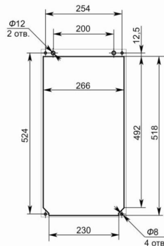
Монтажный вырез утепленный монтаж
