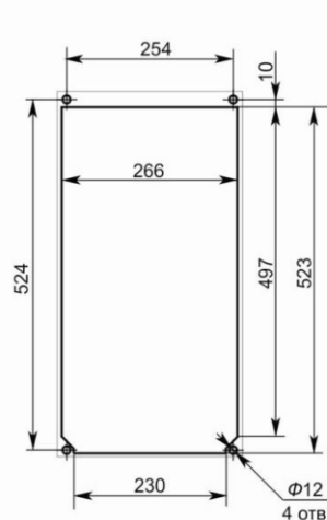
Монтажный вырез полуутепленный монтаж
