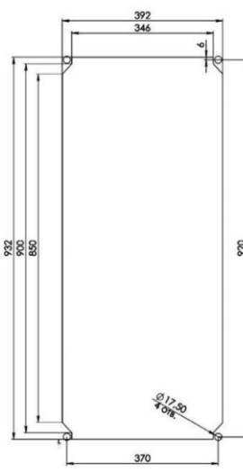
Монтажный вырез полуутепленный монтаж
