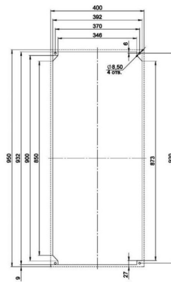
Монтажный вырез утепленный монтаж
