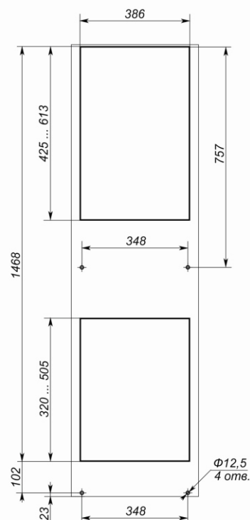
МОНТАЖНЫЙ ВЫРЕЗ наружный монтаж в шкаф глубиной до 500 мм
