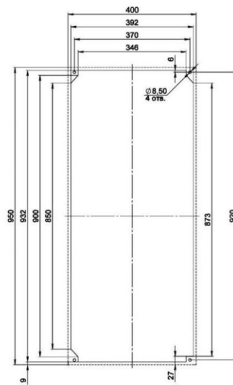
Монтажный вырез утопленный монтаж
