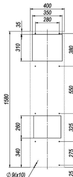
Монтажный вырез наружный монтаж
