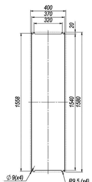
Монтажный вырез полуутепленный утепленный монтаж
