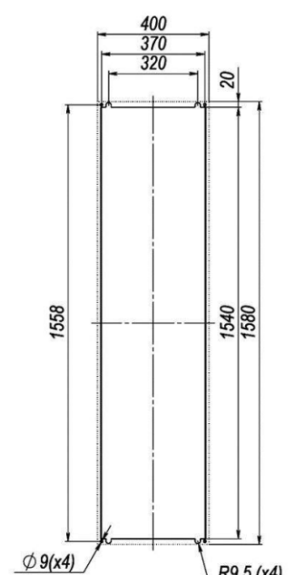
Монтажный вырез полуутепленный, утепленный монтаж
