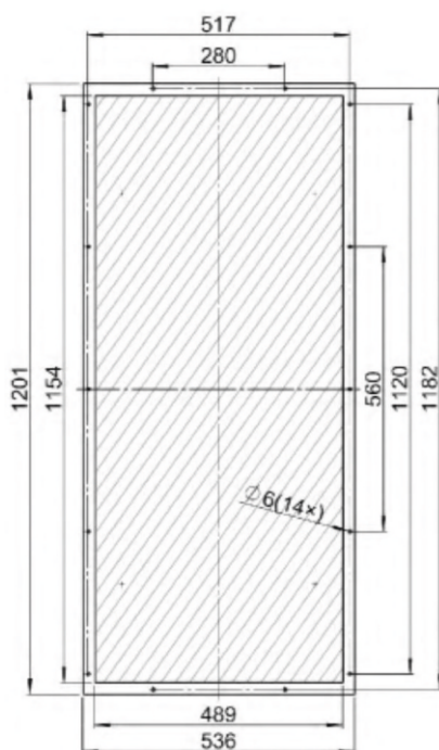
ЧЕРТЕЖИ ПРИСОЕДИНИТЕЛЬНЫХ РАЗМЕРОВ UNISPLIT NS-2500(1)W
