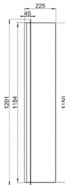
ЧЕРТЕЖИ ПРИСОЕДИНИТЕЛЬНЫХ РАЗМЕРОВ UNISPLIT NS-2500(1)W
