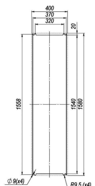
Монтажный вырез полуотопленный, утопленный монтаж
