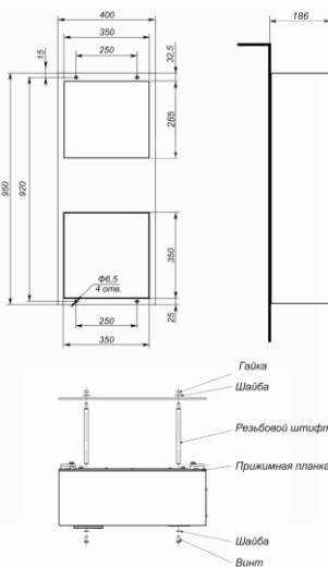
МОНТАЖНЫЙ ВЫРЕЗ наружный монтаж
