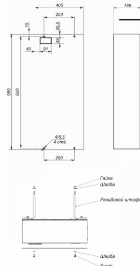
МОНТАЖНЫЙ ВЫРЕЗ утропленный монтаж
