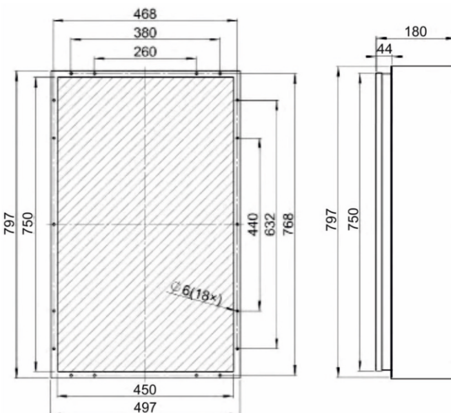
ЧЕРТЕЖИ ПРИСОЕДИНИТЕЛЬНЫХ РАЗМЕРОВ UNISPLIT NS-1000(1)W
